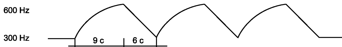
Рисунок 2 - Диаграмма режима изменяющейся тональности
